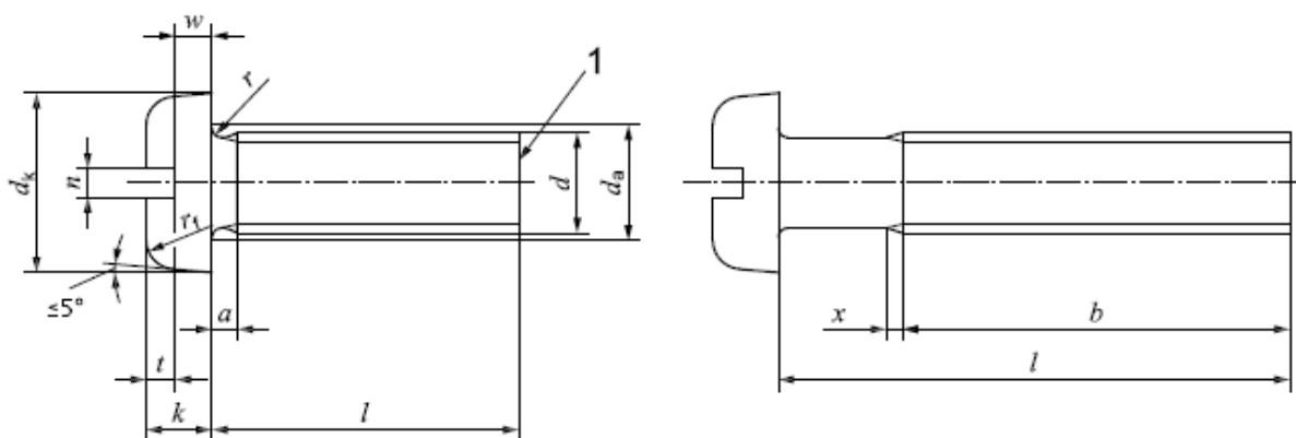
1 Конец без фаски
